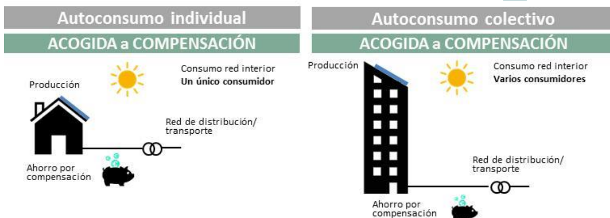
Figura 5: Diagramas de autoconsumo CON excedentes acogidas a compensación
