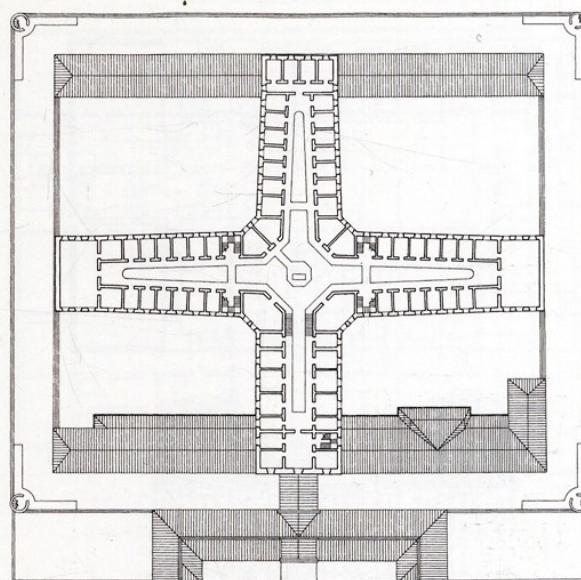
Planimetría orixinal do Cárcere
