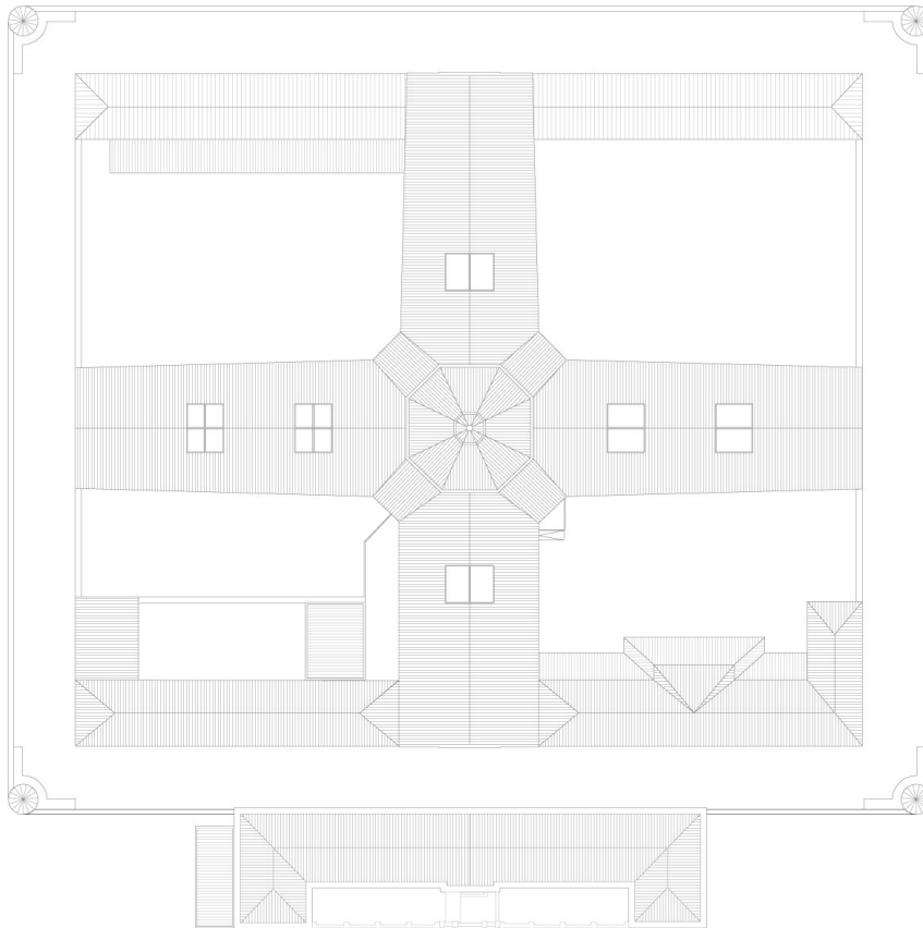
Planta de cubertas
